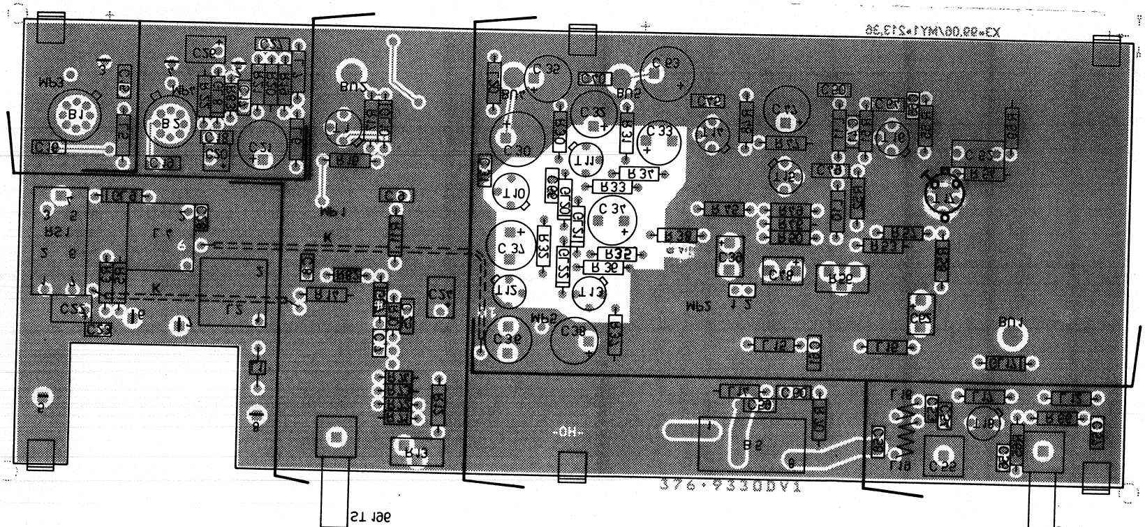
Ansicht und Leitungsführung Lotseite View of tracks on solder side
