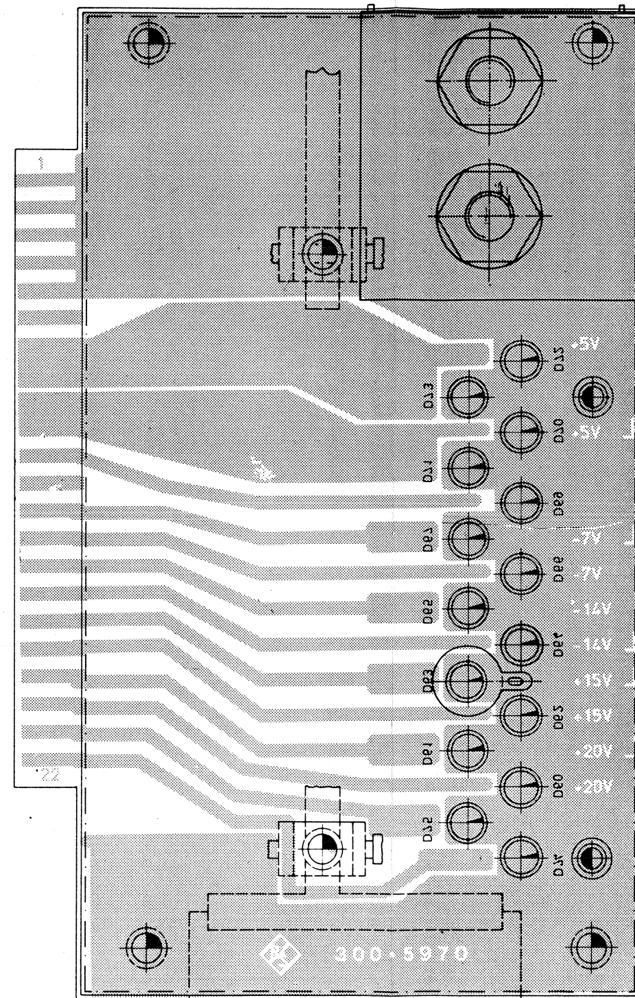
Ansicht und Leitungsführung Lotseite View of tracks on solder side
